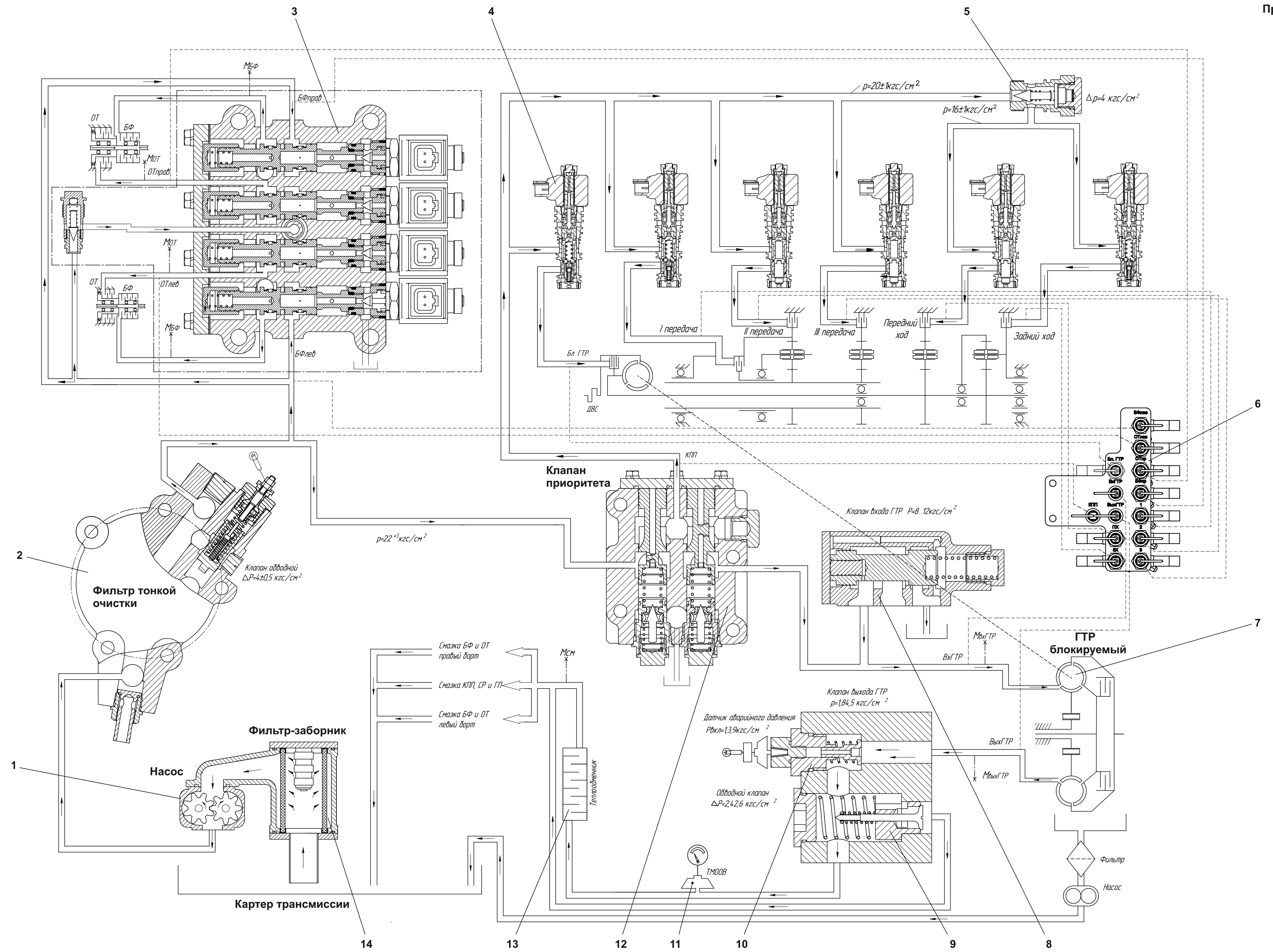
Функциональная схема гидросистемы управления автоматической гидромеханической трансмиссией (лист 2)
