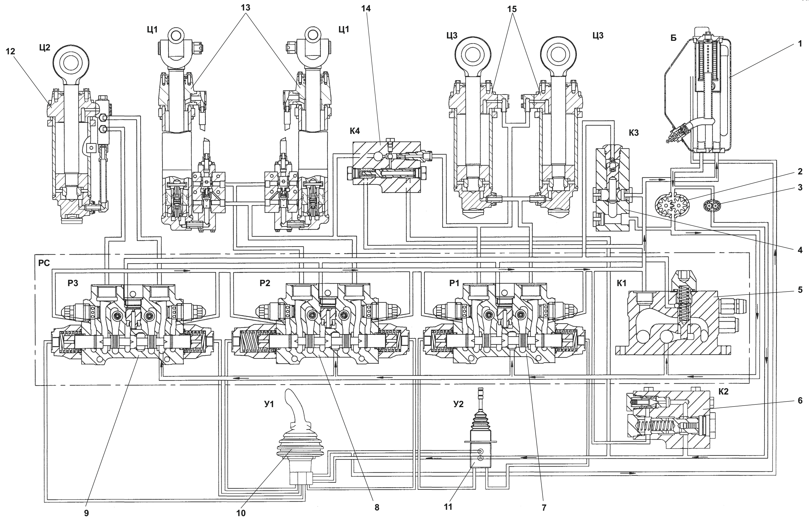
Функциональная схема гидросистемы управления бульдозерным и рыхлительным оборудованием
