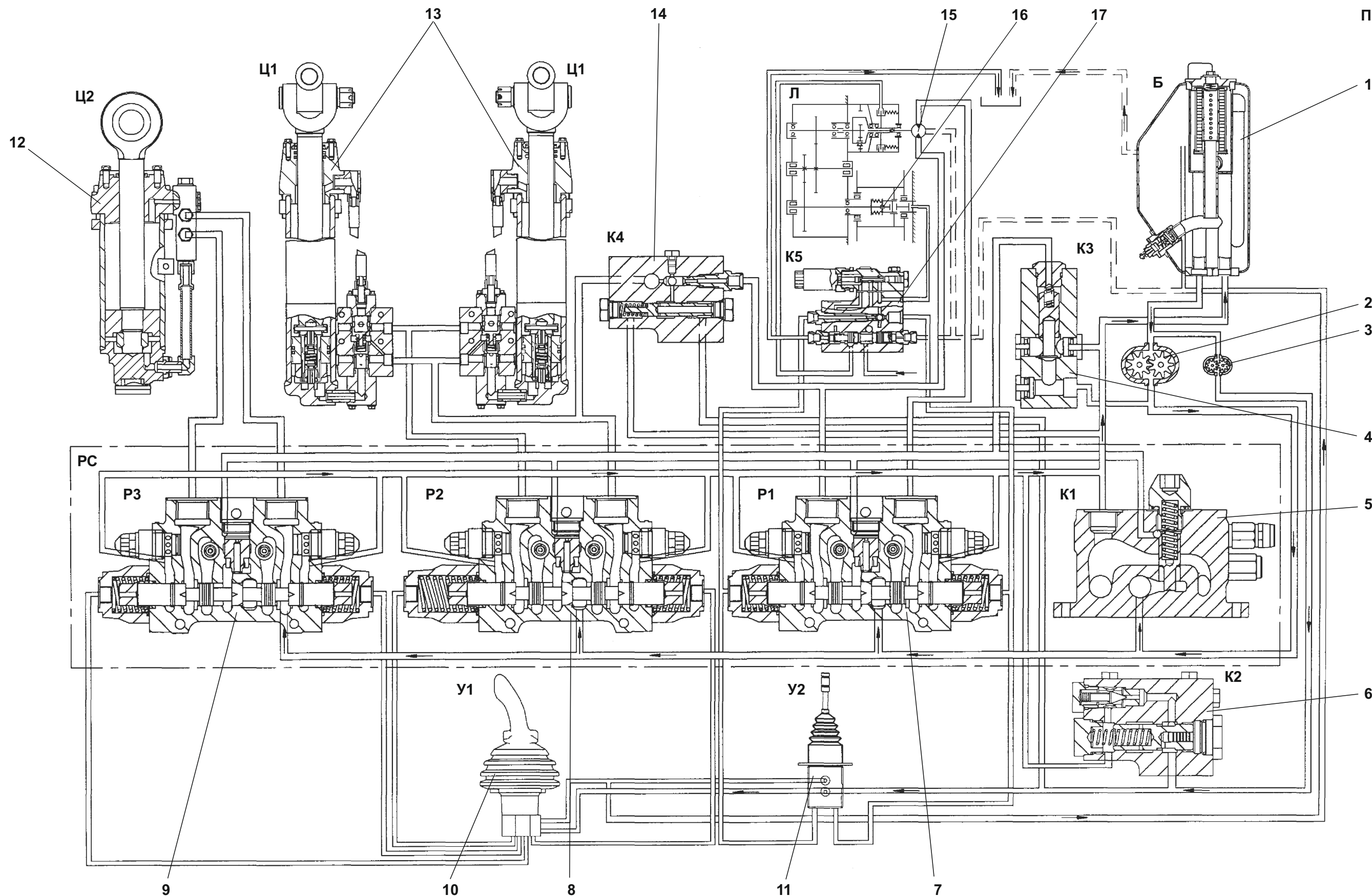
Функциональная схема гидросистемы управления бульдозерным оборудованием и тяговым агрегатом
