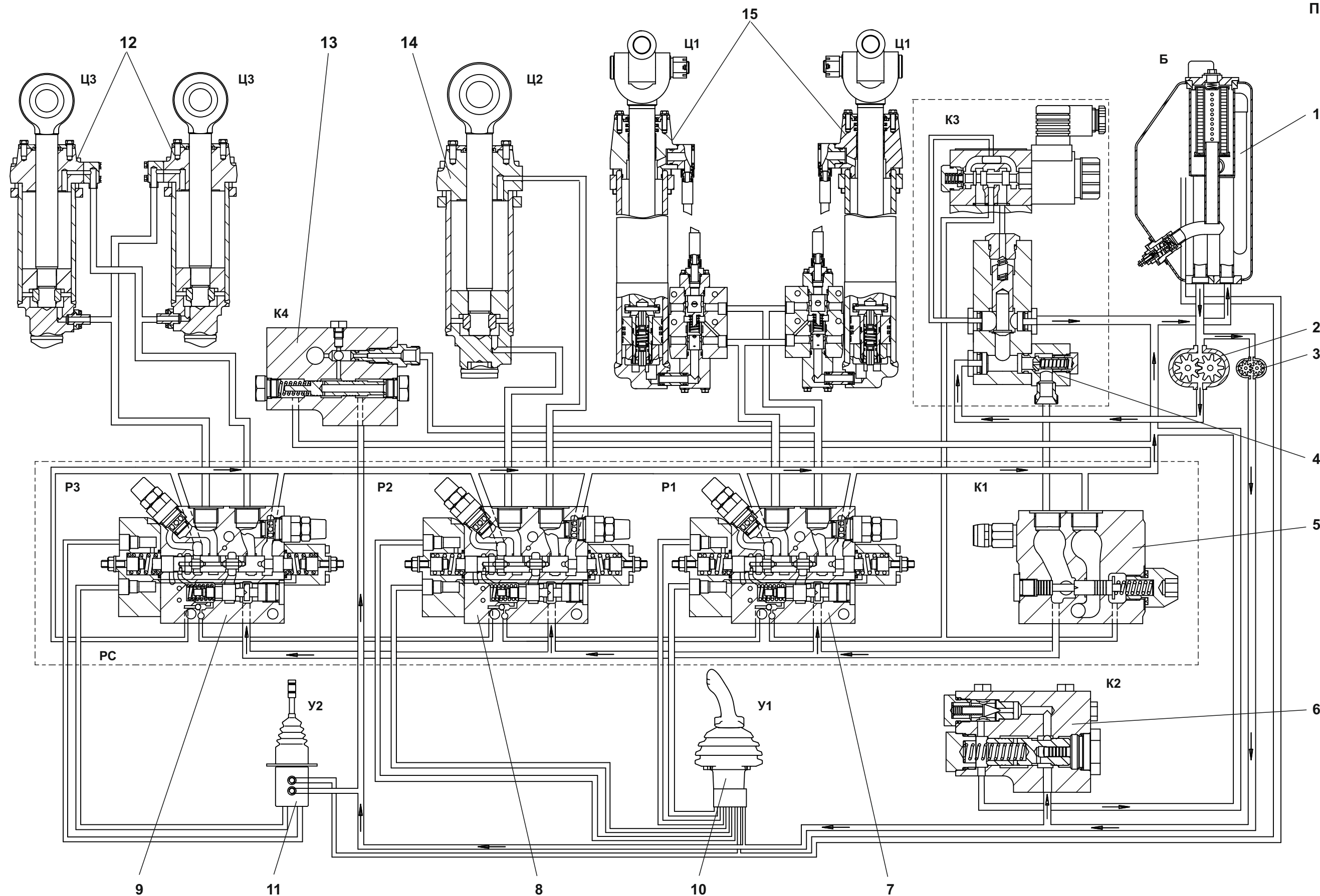
Функциональная схема гидросистемы управления бульдозерным оборудованием бульдозера Т-9.01ЯМП
